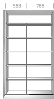
(DYBDE 409 MM) GARDEROBE 1400 MM
